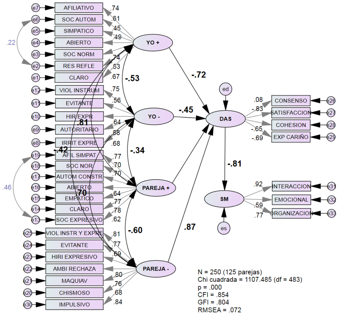
Figura 1. Modelo de ecuaciones estructurales y su bondad de ajuste.
