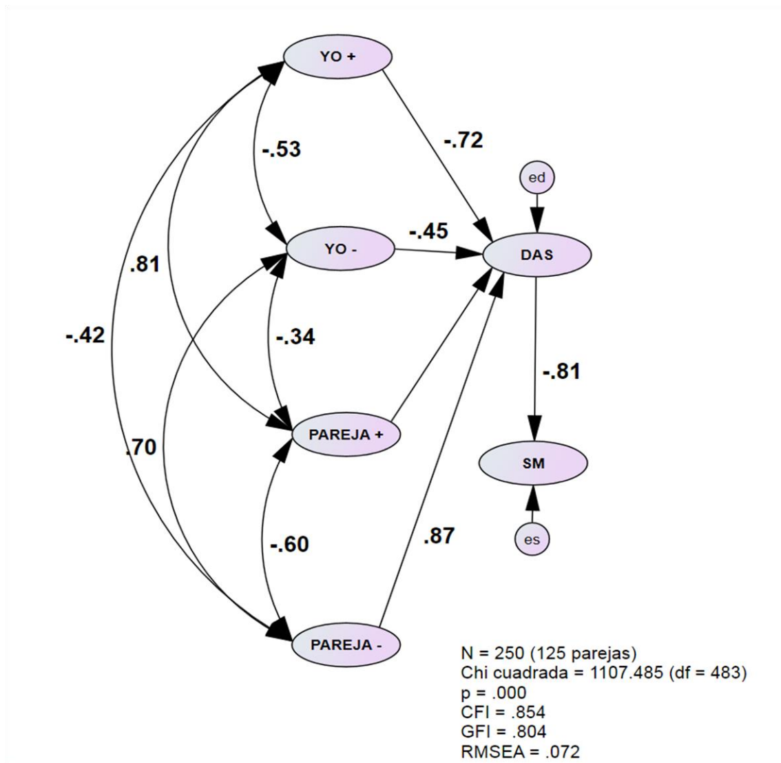
Figura 2. Modelo estructural de las relaciones entre variables latentes.
